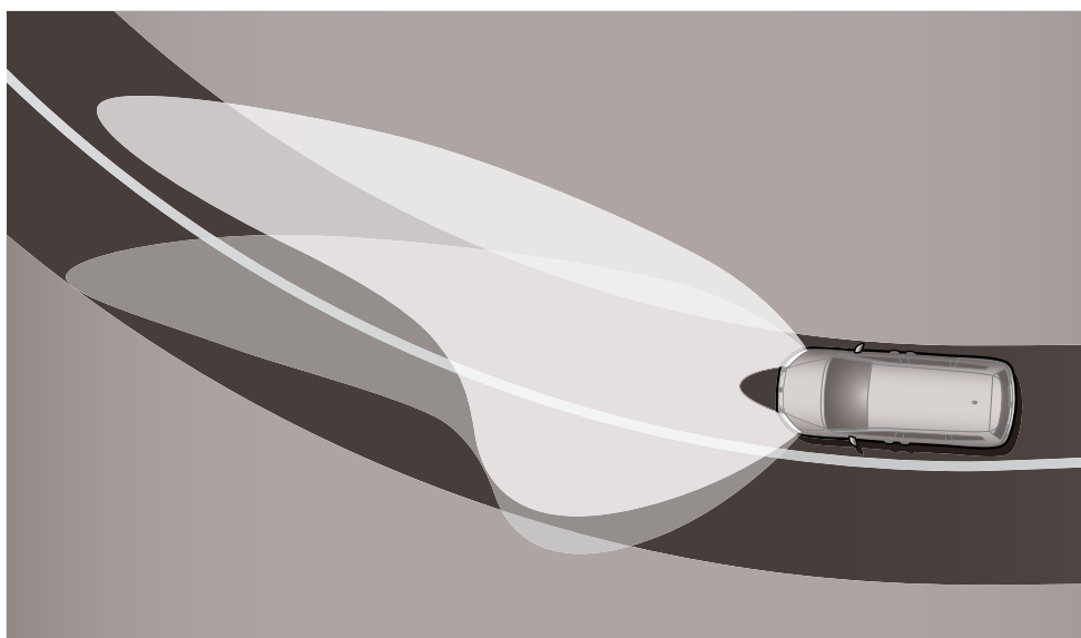
Les phares Bi-Xénon auto-directionnels viennent éclairer l'intérieur des virages en fonction de l'angle du volant.
