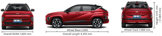
*Unit: mm, data dimensi di atas berdasarkan pada model Signature Long Range. (.) Dengan roof rack.
