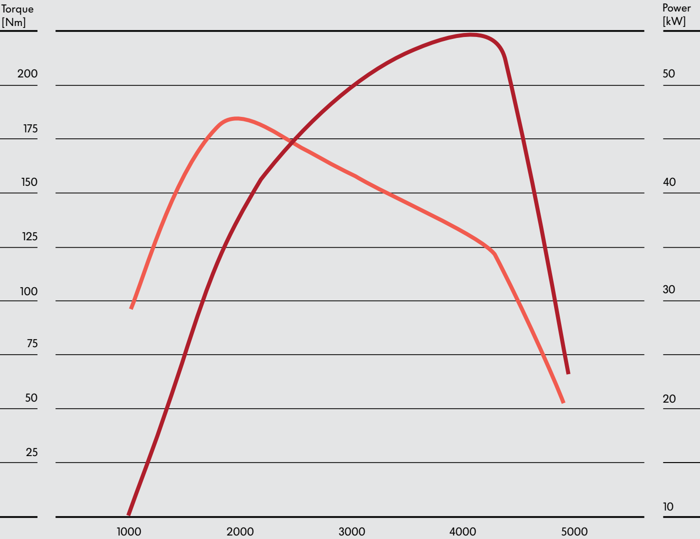
1.2L-75 PS [55 kW] TDI-CR
