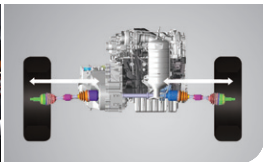
Albero di trasmissione di pari lunghezza per una perfetta stabilizzazione
