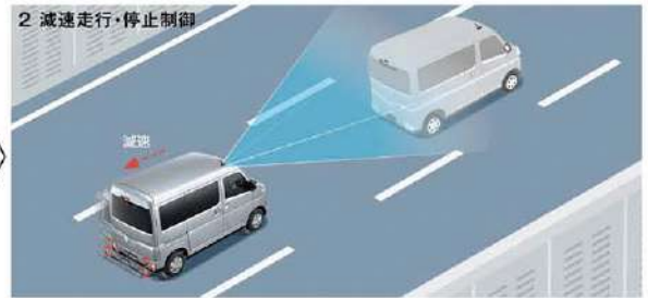
2 減速走行・停止制御 先行車を認識した場合は、先行車の車速に合わせて減速し、先行車が停止すると、先行車に続いて停止します。(停止保持時間は最長約2秒間)
