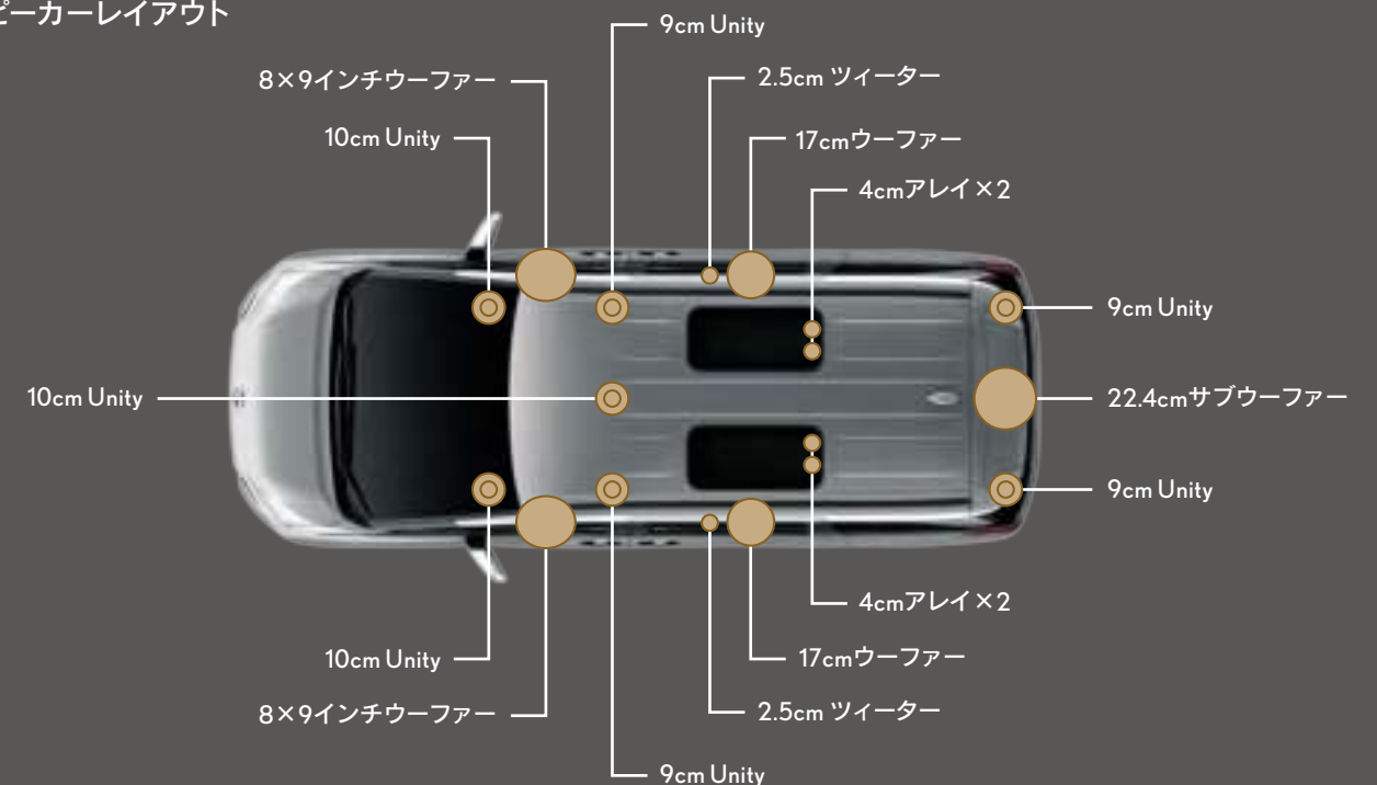
23スピーカーレイアウト
