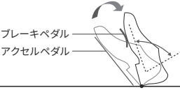
マツダのペダルレイアウト 前輪を前方に移動し、足を自然に伸ばした位置にペダルを配置
