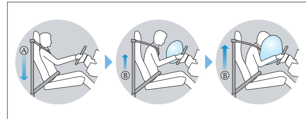
①プリテンショナー（運転席、助手席） ②可変ロードリミッター（運転席、助手席）
