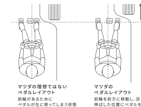
マツダが考える理想のペダルレイアウト
