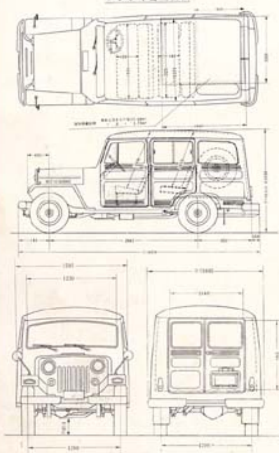
J 30 外觀三视图
