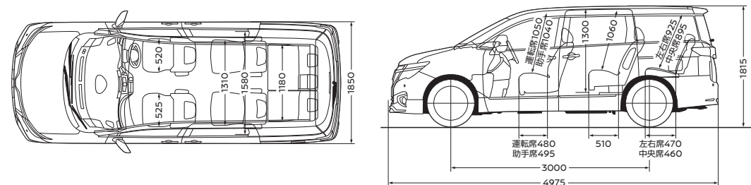
二面図 (250Highway STAR Premium Urban CHROME) 単位: mm
