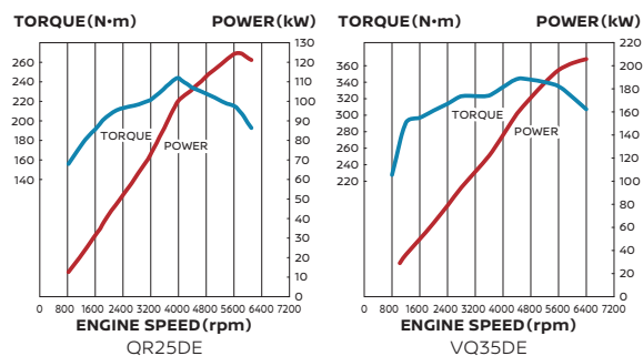
エンジン性能曲線
