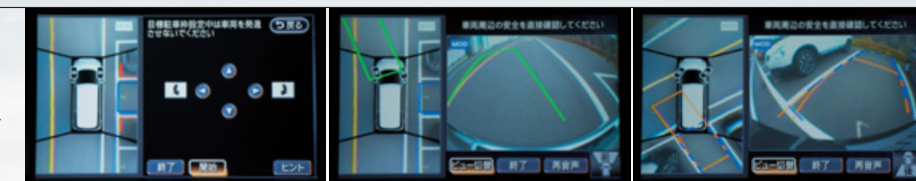
1. 駐車スペース前で停車し、自動認識された目標駐車枠を確認。ガイド開始。 2. 後退開始位置まで前進。 3. 目標進路線に予想進路線が沿うようにステアリングを切り、目標駐車位置まで後退。
