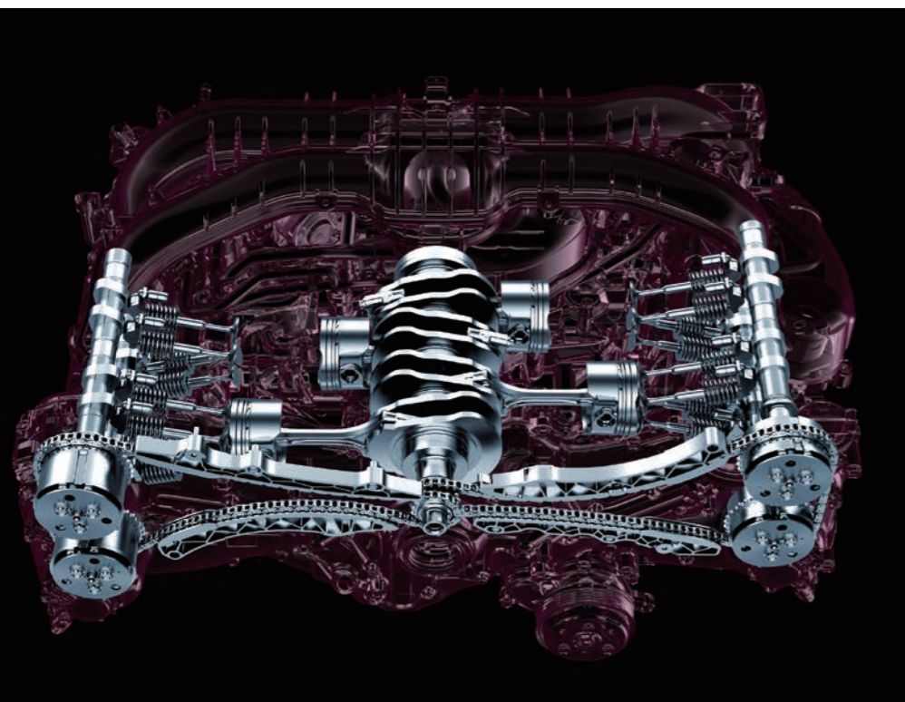
動力性能と環境性能を高次元で両立する2.0ℓ ハイパフォーマンス“DIT”
