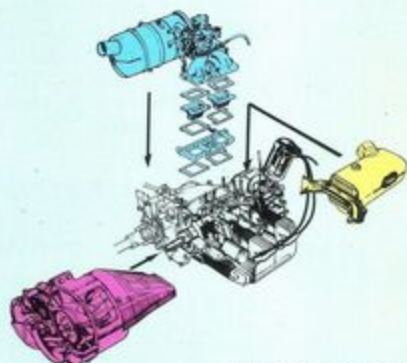
エンジン・ミッション構造図
