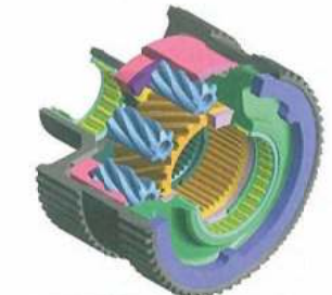
トルセン ® L.S.D.断面図
