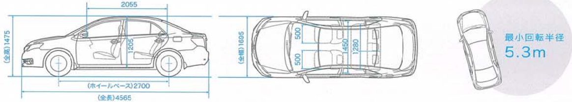
寸法図 (単位: mm) A18 (2WD)
