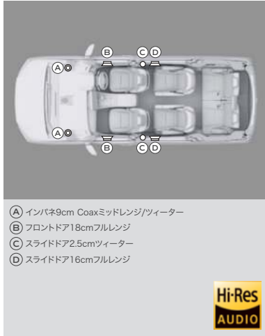
スピーカー配置図
