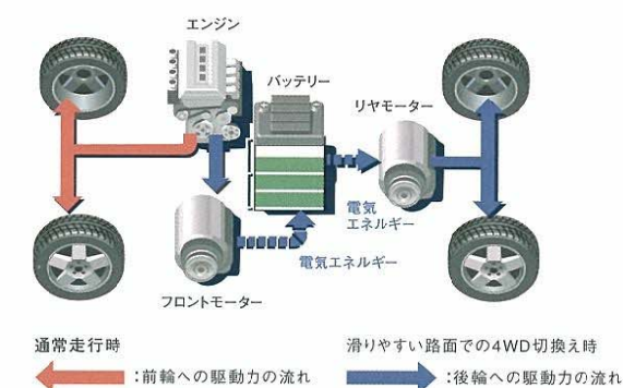
E-Fourシステム図
