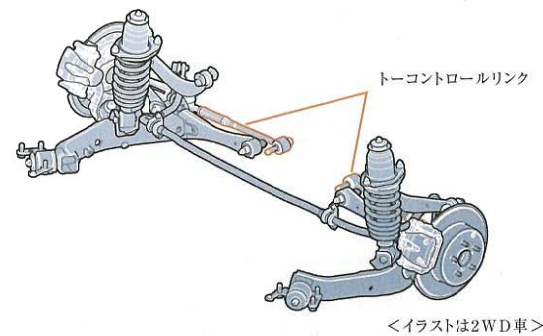
トーコントロールリンク付ダブルウィッシュボーンサスペンション (リヤ)
