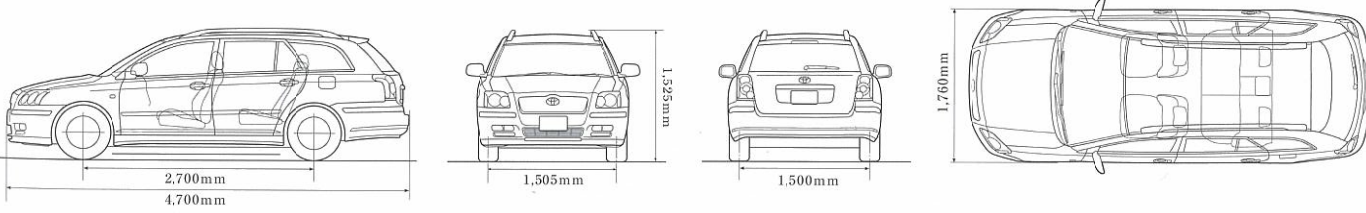
寸法図:ワゴン Li (2WD)
