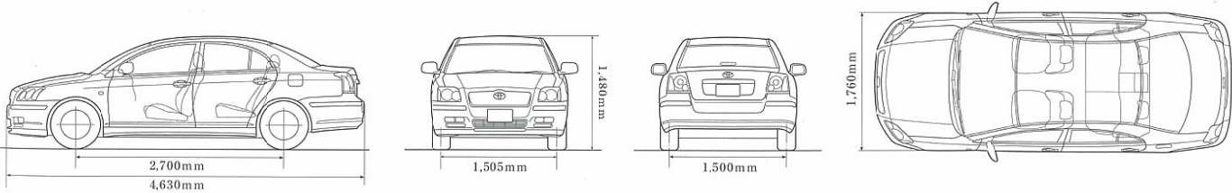
寸法図:セダン Li (2WD)
