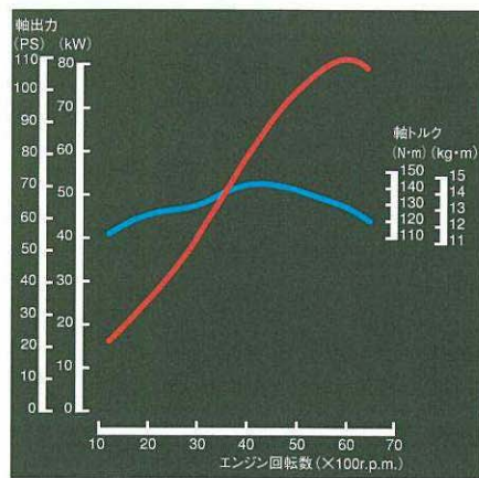
エンジン性能曲線図【1NZ-FE (1.5ℓ)】
