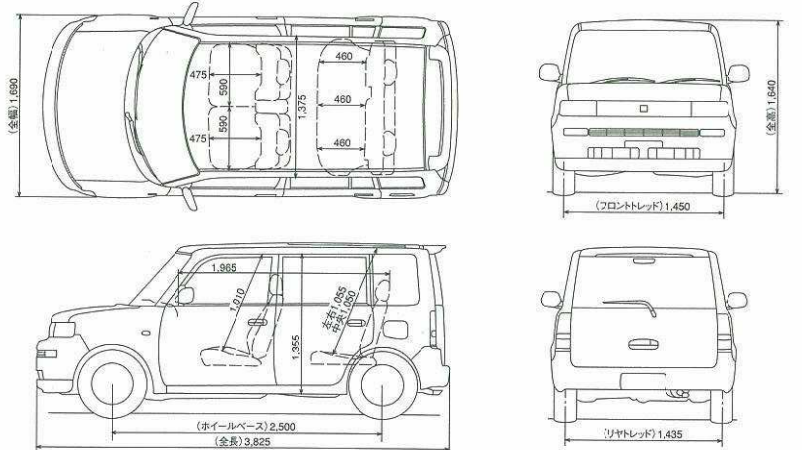
寸法図: トヨタ bB 1.5 Z メーカーオプション装着車 (単位:mm)
