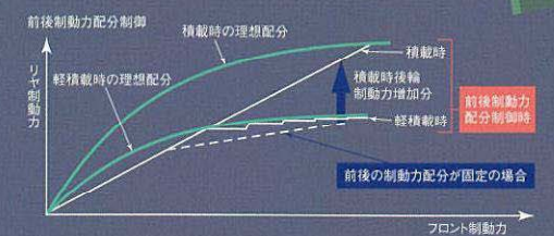
EBD説明図
