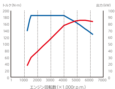
1.2Lターボエンジン性能特性 — トルク — 出力
