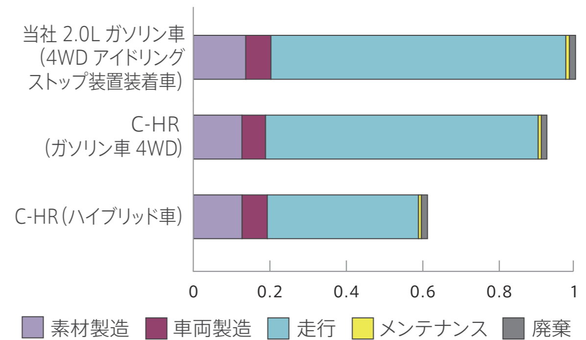
LCA 実施結果 CO 2 二酸化炭素 (Carbon Dioxide)
