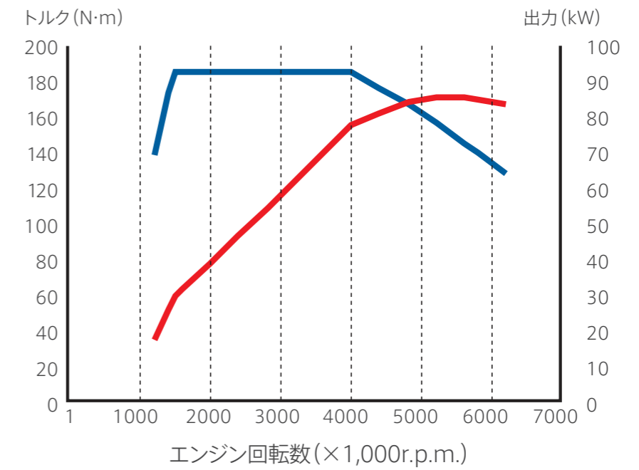
1.2Lターボエンジン性能特性 —トルク—出力
