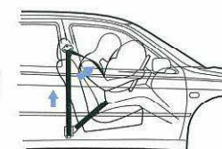
フォースリミッター機構
