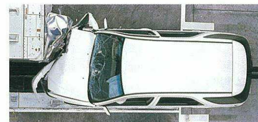
●オフセット前面衝突実験 (64km/h) [写真は実験用の試作車です]
