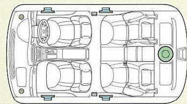
スーパーライブサウンドシステム・スピーカー配置図 ●ダッシュボードホーンツイーター ●ウーハー ●ドアスピーカー ●ドアツイーター
