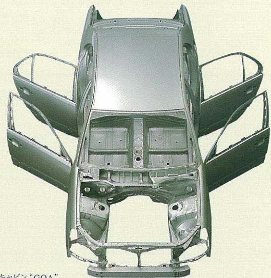
衝撃吸収ボディ&高強度キャビン“GOA”
