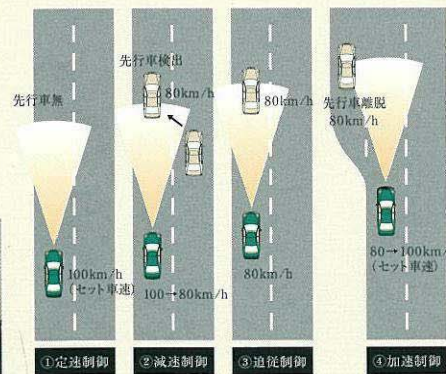
①定速制御 ②減速制御 ③追従制御 ④加速制御
