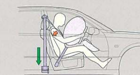
プリテンショナー機構
