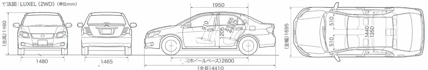
寸法図: LUXEL (2WD) (単位:mm)
