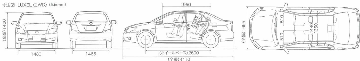
寸法図:LUXEL(2WD)(単位:mm)
