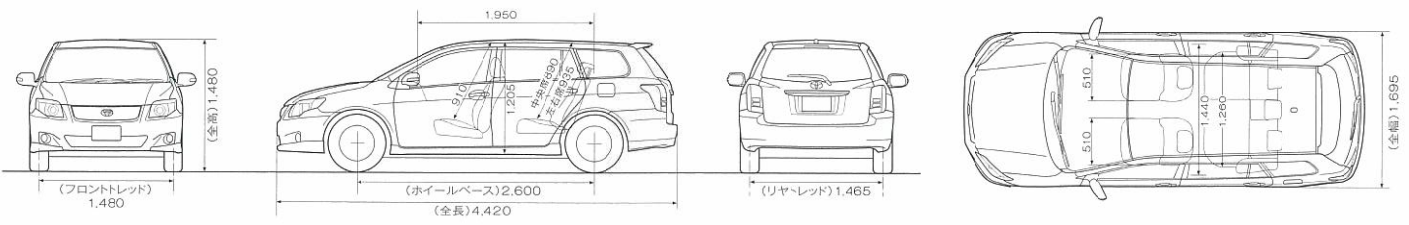
寸法図：トヨタ カローラ フィールダー 1.8S "AEROTOURER" 2WD(単位mm)
