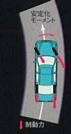
左右制動力配分制御
