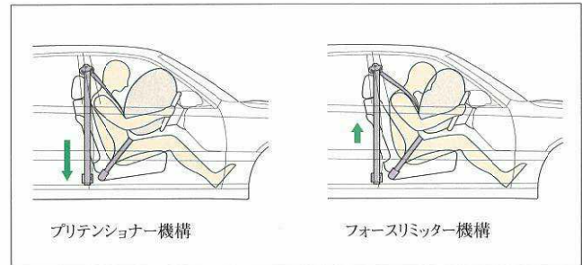
プリテンショナー&フォースリミッター機構
