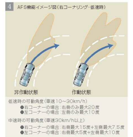
4 AFS機能イメージ図(右コーナリング・低速時)
