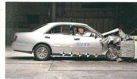
オフセット前面衝突実験(64km/h、写真は実験用試作車です。)
