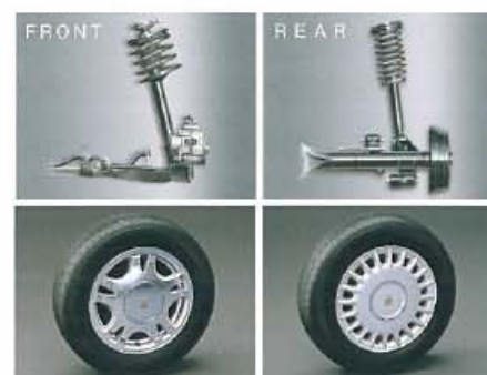
FRONT REAR 195/65R15 91H 51 2JJ 195/65R15 91S 51 2JJ アルミホイール+センターオーナメント スチールホイール+樹脂フルキャップ
