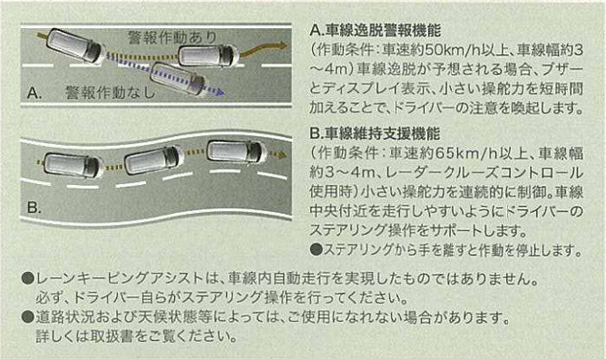
■レーンキープアシスト(LKA)
