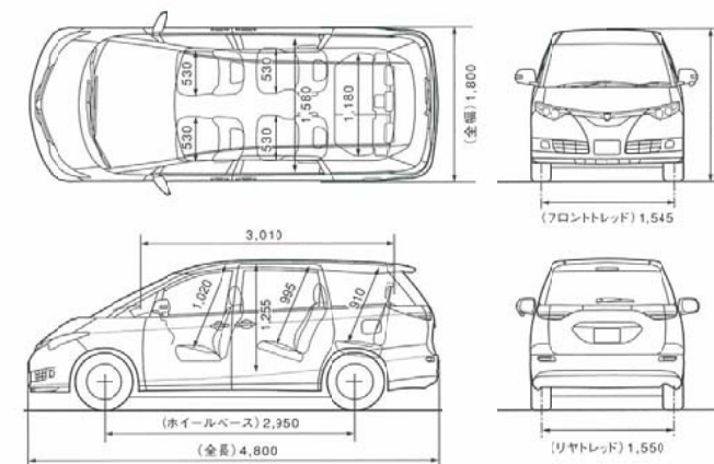
寸法図：エスティマハイブリッド(7人乗り) (単位:mm)
