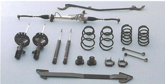
エアラス-S専用サスペンション
