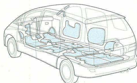
遮音材・吸音材配置図
