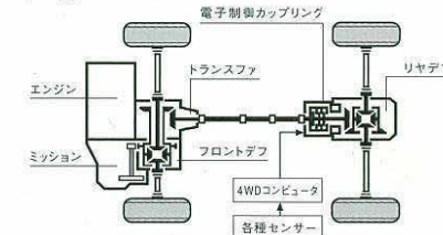
システム図
