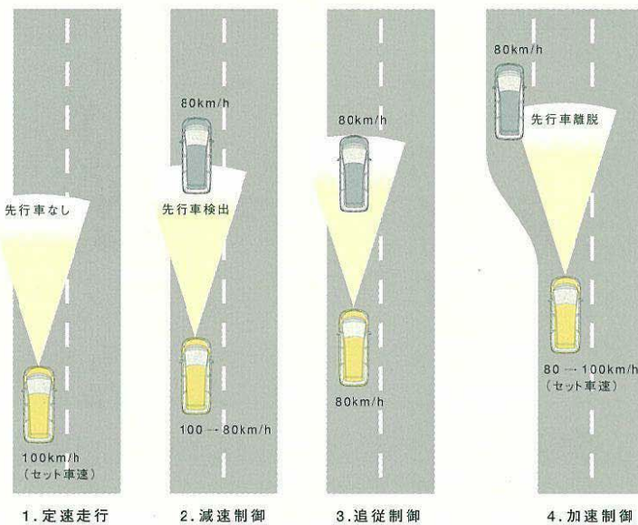
レーダークルーズシステムの典型的な動作例
