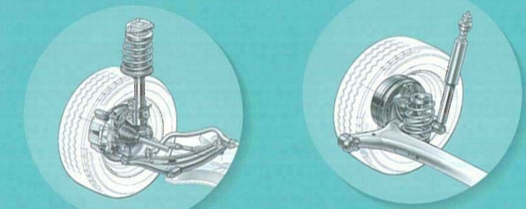
フロント:Lアーム式マックファーソンストラット式サスペンション リヤ:イータビームサスペンション(トールコイル機能付トーションビームサスペンション)
