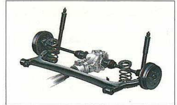
トーションビーム式コイルスプリングサスペンション (イラストはリヤ・4WD)
