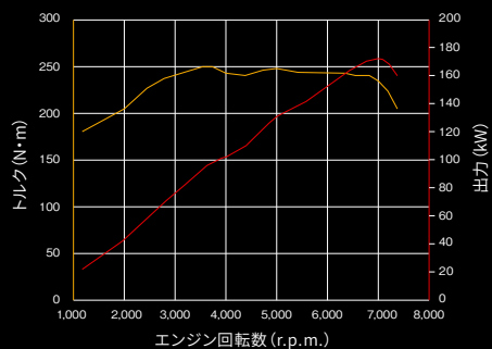
■エンジン性能曲線図
