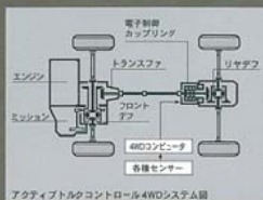
アクティブトルクコントロール4WDシステム図
