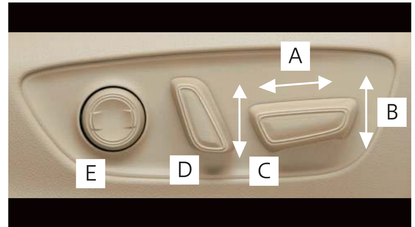
□A前後スライド □B座面前端上下 □Cシート上下 □Dリクライニング □Eランバーサポート
