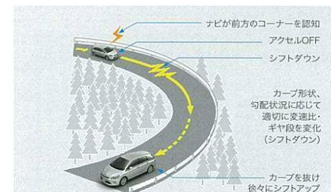
コーナー走行時作動例
