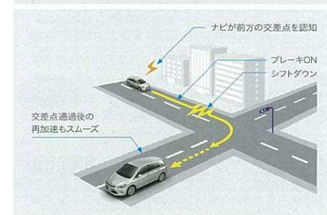
交差点走行時作動例 (経路案内中のみ実施)
