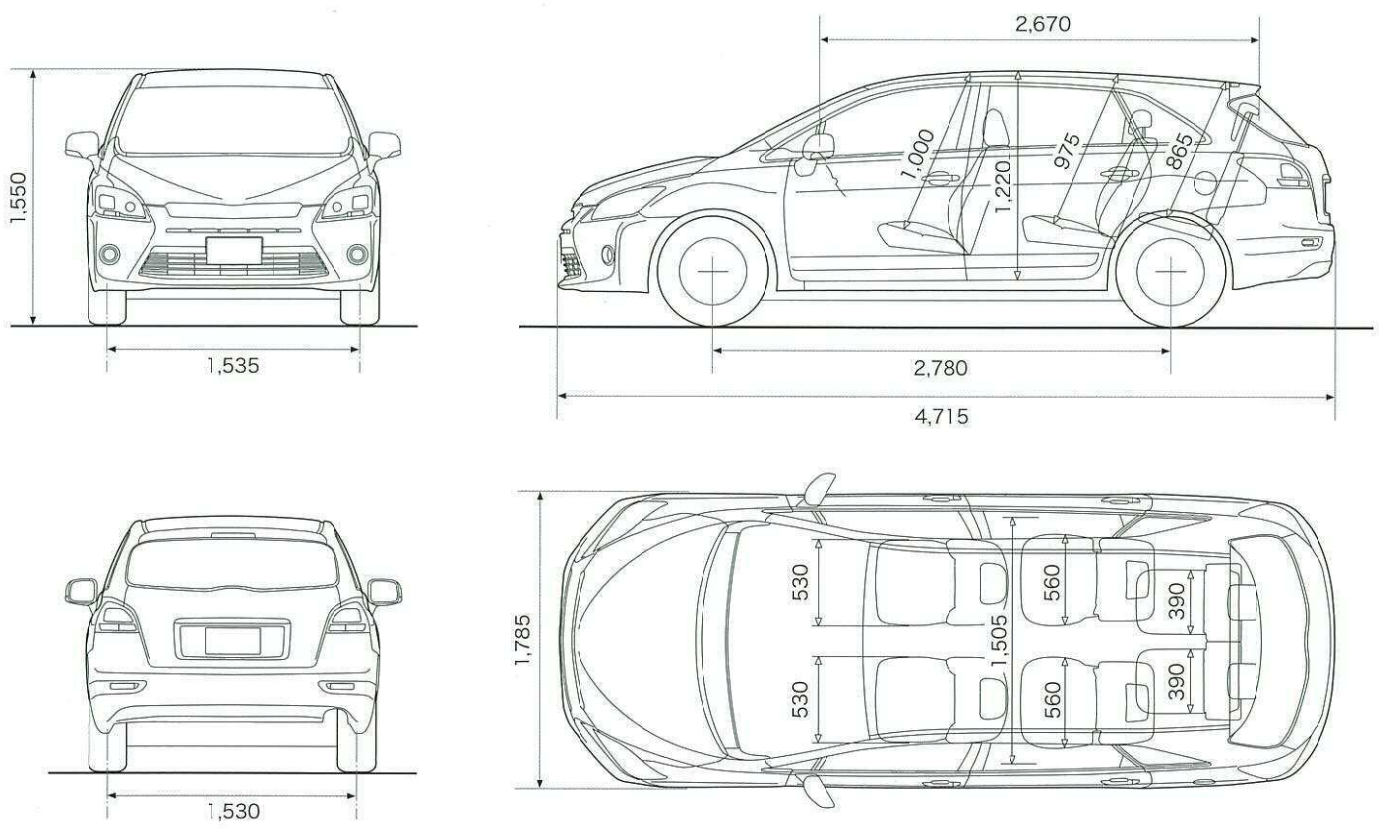
寸法図:トヨタ マークXジエ 240G(2WD・6人乗り)(単位mm)
