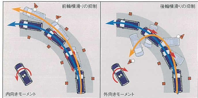
VSC説明図
