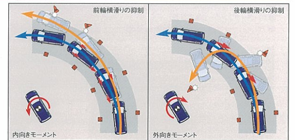
VSC説明図
