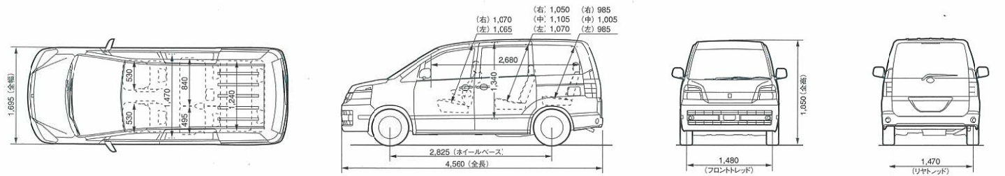
■トヨタ ヴォクシー Z 寸法図
