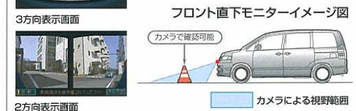
フロント直下モニターイメージ図 カメラによる視野範囲
