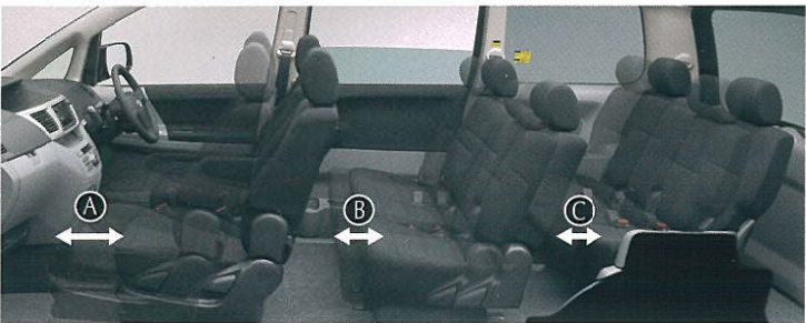
A:スライド量:225mm (運転席・助手席) B:スライド量:180mm (セカンドシート・マルチ回転シートの場合) 105mm (ワンタッチタンブルシートの場合) C:スライド量:155mm ※TRANS-Xはシートスライドしません。
