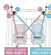
左右席同時定位原理図
