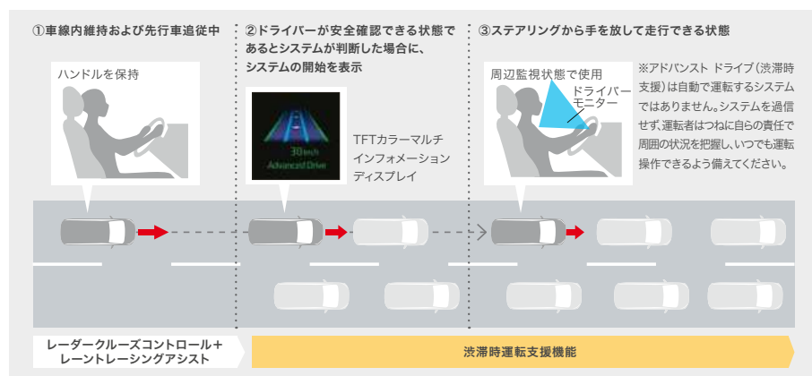
ドライバーモニターカメラ ■ドライバーモニターカメラで運転者の顔の位置・向きや眼の開閉状態を検知。運転者が周囲の状況を確認し運転操作できる状態であるかシステムが判断し、ブザーとディスプレイ表示で注意喚起を行います。 *3
