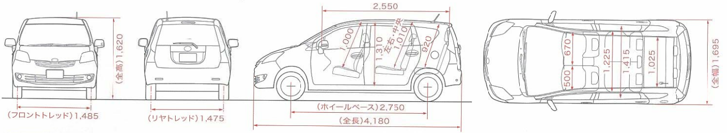
寸法図：トヨタ パッソ セッテ G “C Package” (2WD) 単位(mm)
