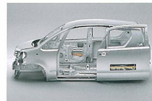
衝撃吸収ボディ&高強度キャビン“GOA”
