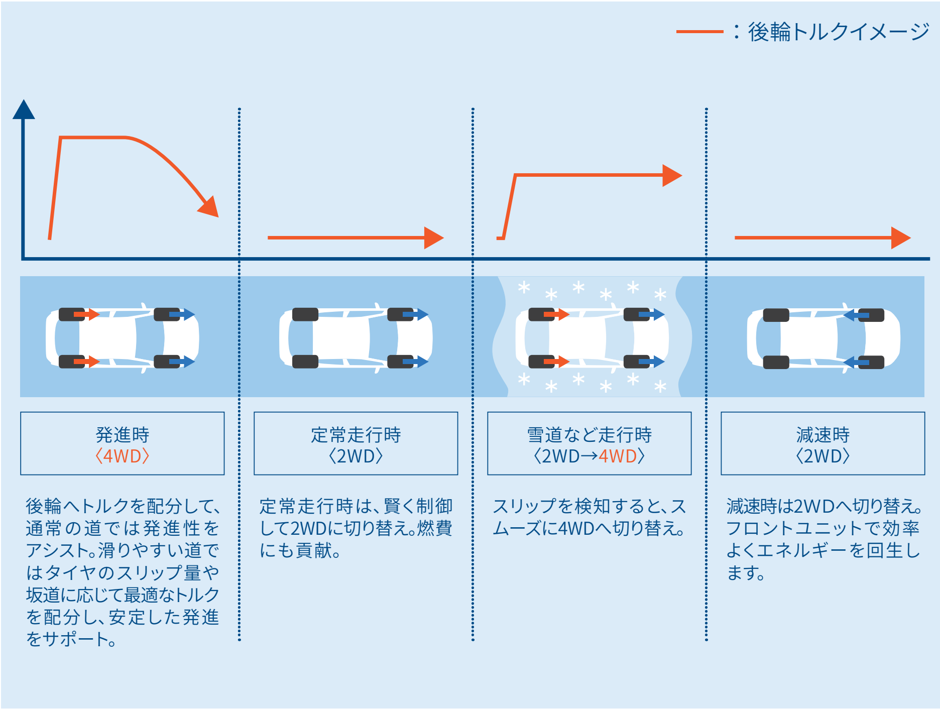
前後輪トルク配分イメージ
